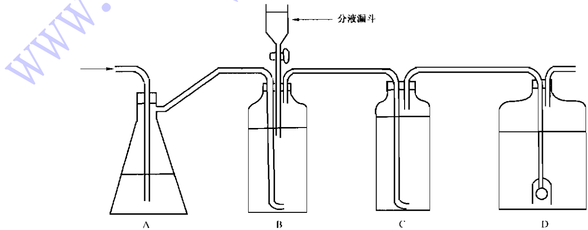
图 1 二氧化氯发生及吸收装置
